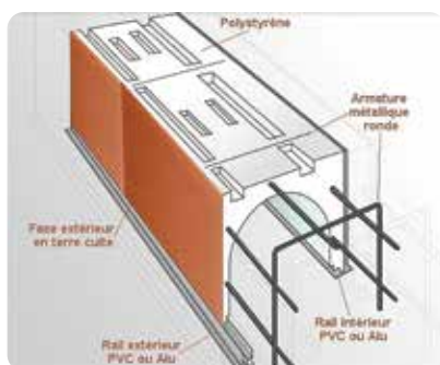
Caisson parement BRIQUELITE
