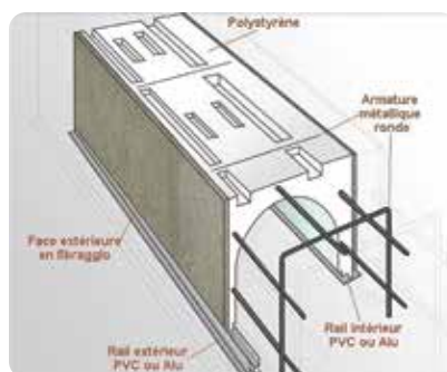
Caisson THERMICOFFRE et THERMIBRIQUE
